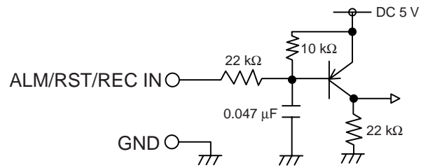
<Schnittstellen-Schaltung im VCR>
