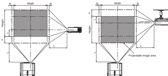
Weitwinkel 22 mm (0,8:1) on-axis
